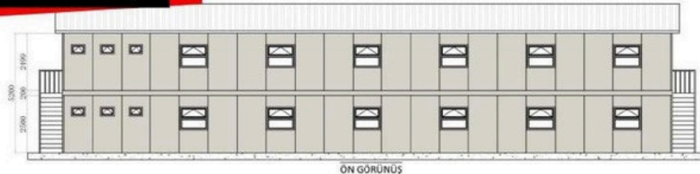
ÖN GÖRÜŞ
