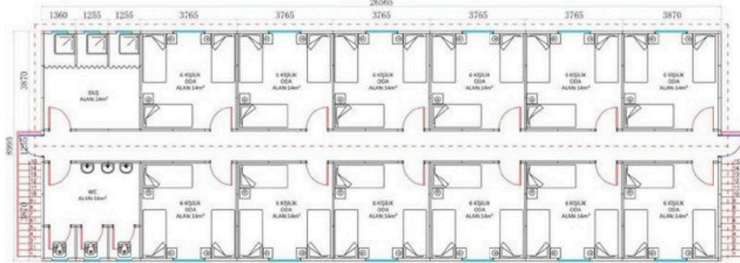
1. KAT PLANI
